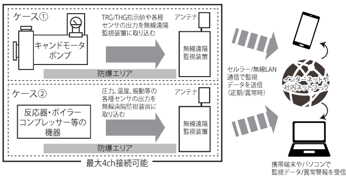
「テイコクモータポンプ無線遠隔システムTRM-W」の通信イメージ図
