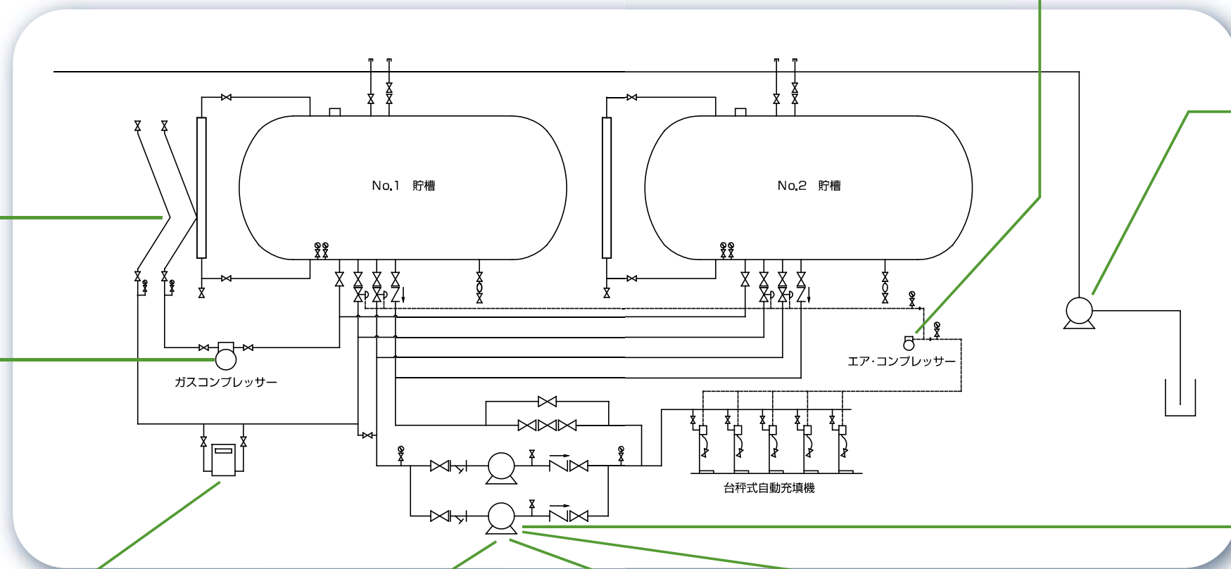
●TBニイガタローディングアーム ローリーからストレージタンクへの受け入れ
