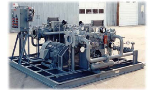
●コーケンガスコンプレッサー
